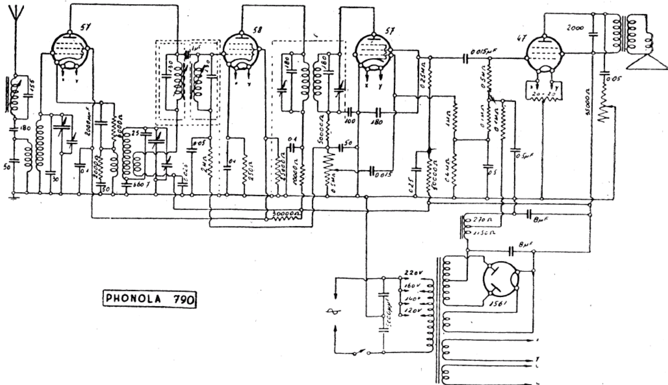
PHONOLA-RADIO (S. A. FIMI). — Modelli: « 790, 791, 792 e 793 ». - Produzione 1935 - Media frequenza: 470 kHz.
